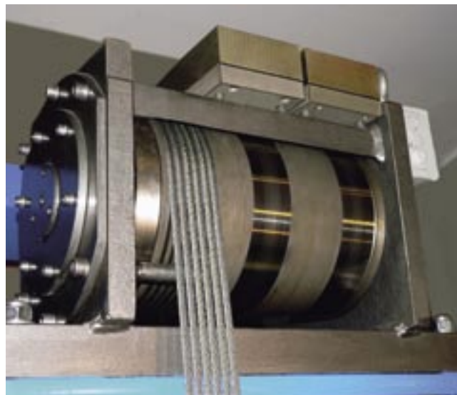
Permanentmagnet-Kompaktantrieb, getriebelos
