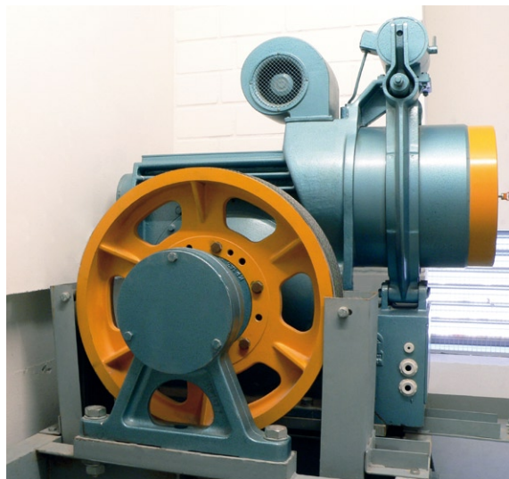
Seilantrieb im Maschinenraum über dem Schacht
