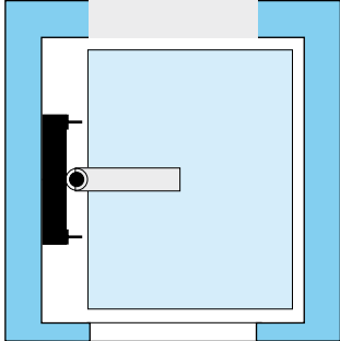
1 Hydraulik-Kolben, seitlich angeordnet (Rucksack-Aufhängung), seitlich geführt
