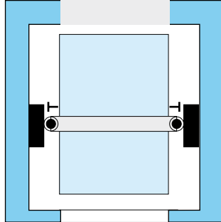
2 Hydraulik-Kolben, beidseitig angeordnet, mittig geführt mit gegenüberliegenden Führungsschienen
