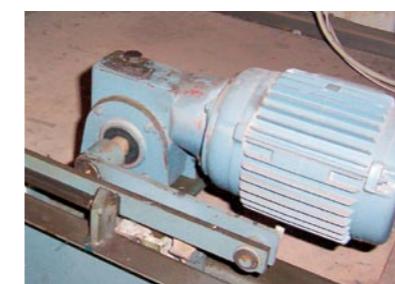
Alter Kabinentürantrieb
