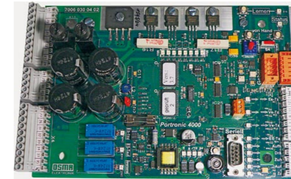
Die von OSMA entwickelte Mikroprozessor-Türsteuerung Portronic 4000
